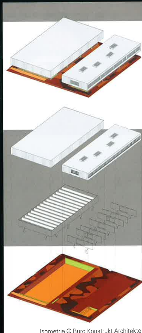
Isometrie © Büro Konstrukt Architekten
